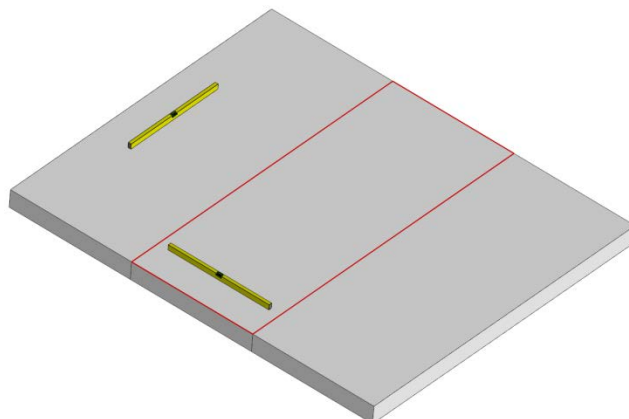
Рисунок 3 – Установка плит с уровнем
