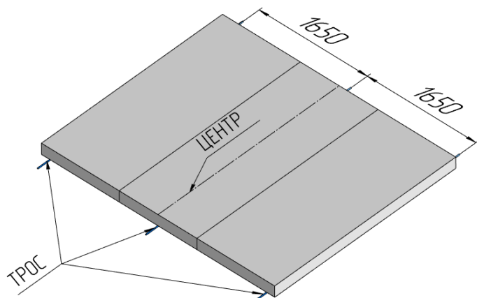
Рисунок 2 – Закладка тросов
