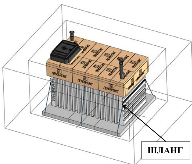
Рисунок 4 – Установка погреба
