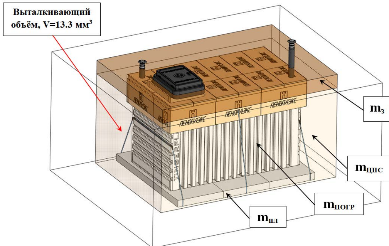
Рисунок 11 – Расчет якорения погреба
