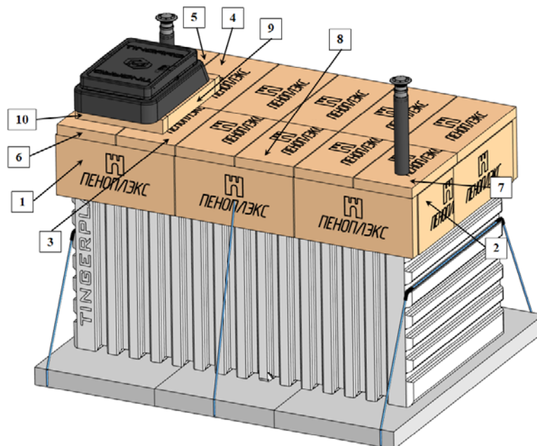
Рисунок 8 – Схема монтажа утеплителя
