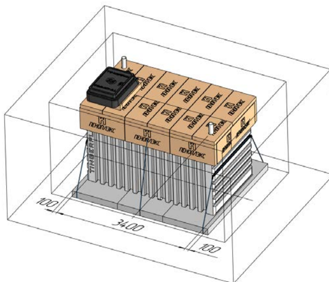
Рисунок 5 – Утепление погреба и закрепление тросами
