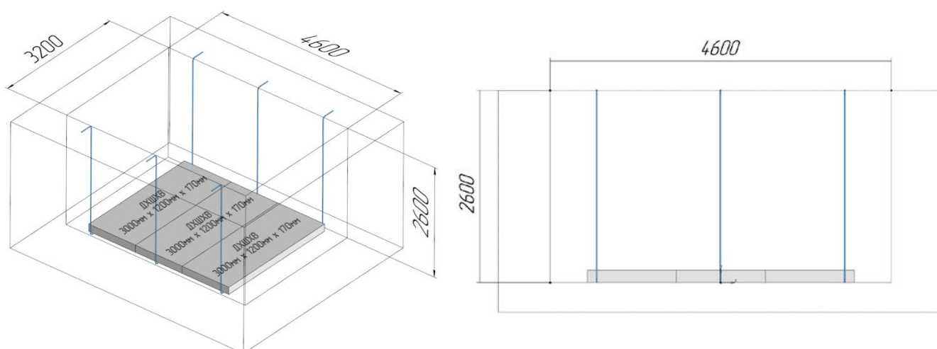
Рисунок 1 – Размеры котлована под установку плит
